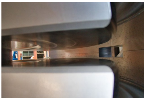
Dans l'entrefer d'un électroaimant
